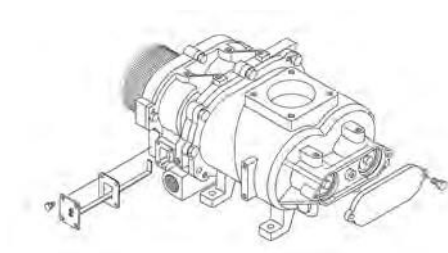
Рис. 57: Выталкиватель для типа 15 – 30
