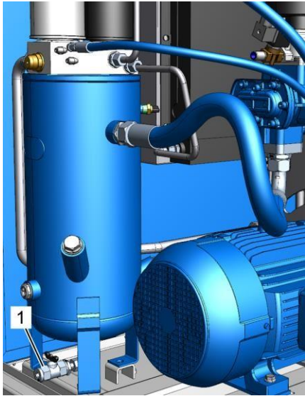
Рис. 42: Отверстие для слива охлаждающей жидкости
